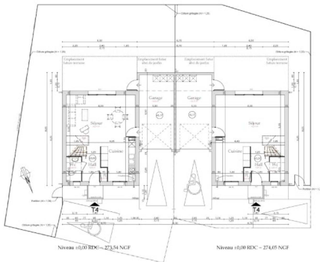
Plan de niveau RDC
